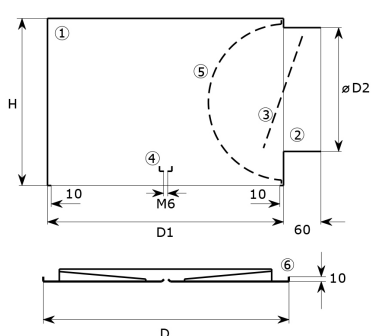
Vrtnični difuzor BD-4
